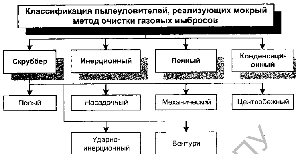
Рис.8.2. Классификация мокрых пылеуловителей
