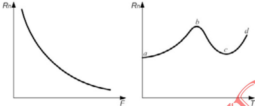
Рисунок 1 – Зависимость переходного сопротивления от силы контактного нажатия (а) и температуры (б)
