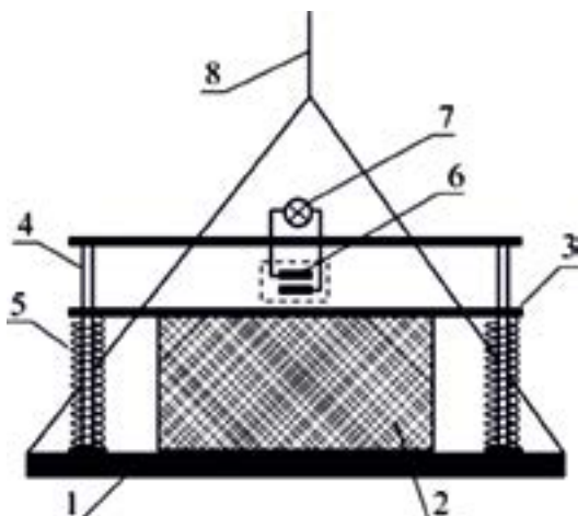
Рисунок 1 – Прибор для дэманстрацыі стану бязважкасці
