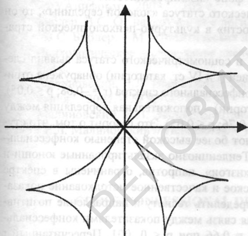
Рис. 2. Функциональный комплекс-фрейм
