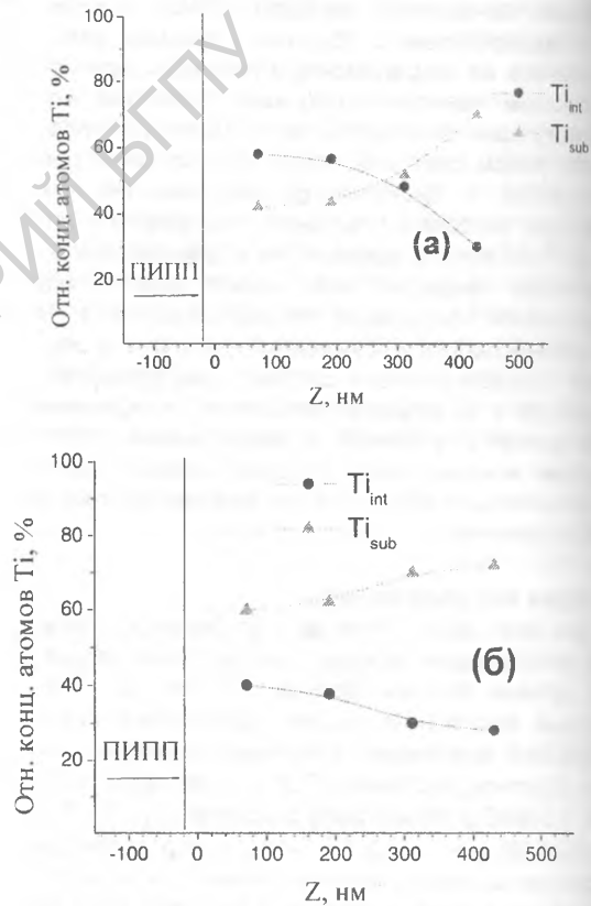
Рис. 3. Распределение в кремнии атомов титана, находящихся в междоузлиях и замещающих положениях кристаллической решетки кремния, в структурах Ti покрытие/Si, сформированных: (а) – методом ОПАСИ, б) – методом ОПАСИ на кремнии, предварительно облученном ионами Хе с энергией 20 кэВ и интегральным потоком 9×10 14 Хе/см 2 .
