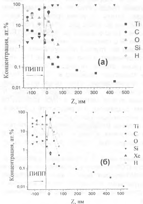
Рис. 1. Распределение атомов титана в кремнии в структурах Ti покрытие/Si, сформированных: (а) – методом ОПАСИ, б) – методом ОПАСИ на кремнии, предварительно имплантированном ионами Хе с энергией 20 кэВ и интегральным потоком 9 \times 10^{14} Хе/см 2
