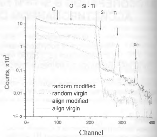
Рис 2. Энергетические спектры POP ионов He + с E 0 =2 МэВ от (100) Si, модифицированного нанесением титанового покрытия методом ОПАСИ предварительно имплантированным ионами Хе с энергией 20 кэВ и интегральным потоком 9×10 14 Хе/см 2 , и исходного (100) кремния.
