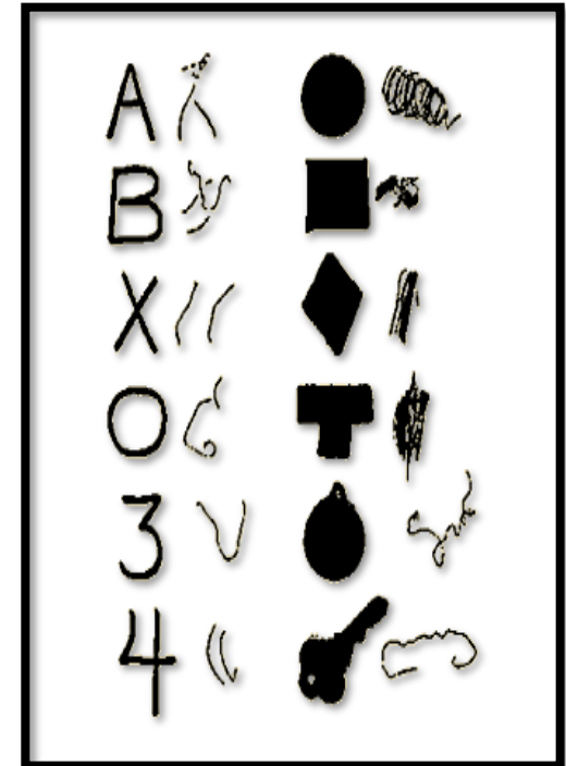
Сімвалічная агназія
