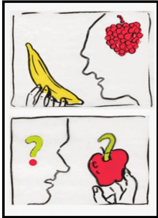
Прадметная агназія
