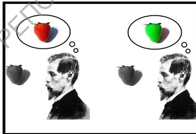
Колеравая агназія
