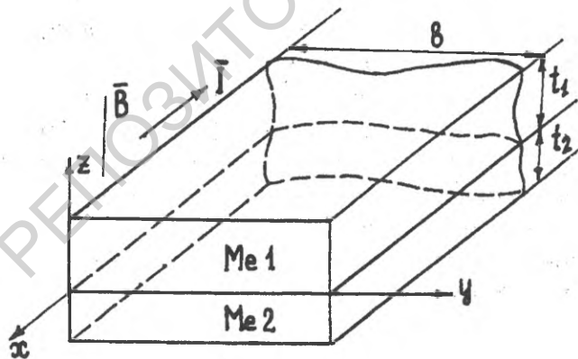
Рис. 1. Пластина́тый композиционный проводник из двух элементов (Me1 и Me2) различной толщины и его ориентация относительно магнитного поля
