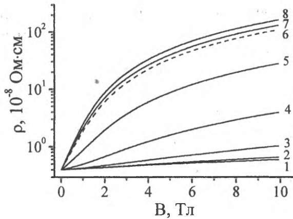
Рис. 2. Сопротивление гипотетического композиционного Al^+-Al^- проводника: величина насыщающейся части сопротивления \rho_s = 4 \cdot 10^{-9} Ом·см; толщина элемента t = 0.5 см; ширина b , см: 5 \cdot 10^{-6} (1), 5 \cdot 10^{-5} (2), 5 \cdot 10^{-4} (3), 5 \cdot 10^{-3} (4), 5 \cdot 10^{-2} (5), 0.5 (6), 1 (7), 1000 (8)
