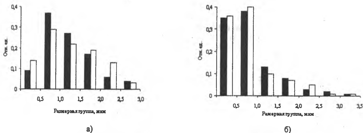
Рис. 2. Распределение частиц твердого раствора на основе \beta -Sn фольг припоев № 1 (а) и № 2 (б) в исходном состоянии по размерным группам
