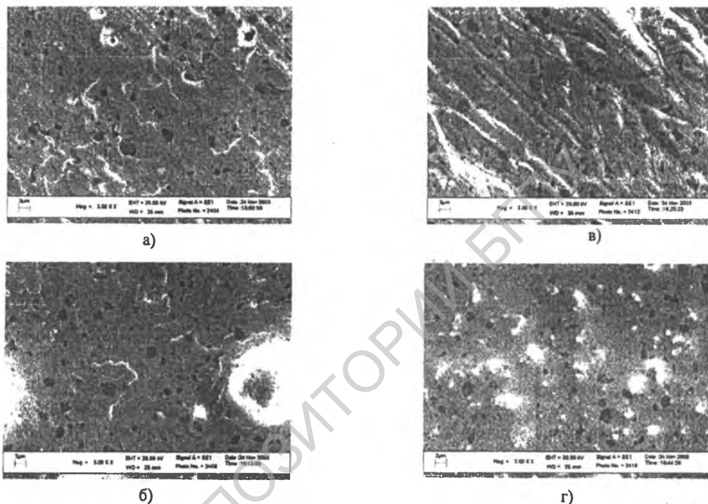
Рис. 1. Микроструктура быстрозатвердевших фольг припоев № 1 (а, б) и № 2 (в, г): а, в – сторона фольги, прилегающая к кристаллизатору; б, г – сторона фольги, контактирующая с атмосферой
