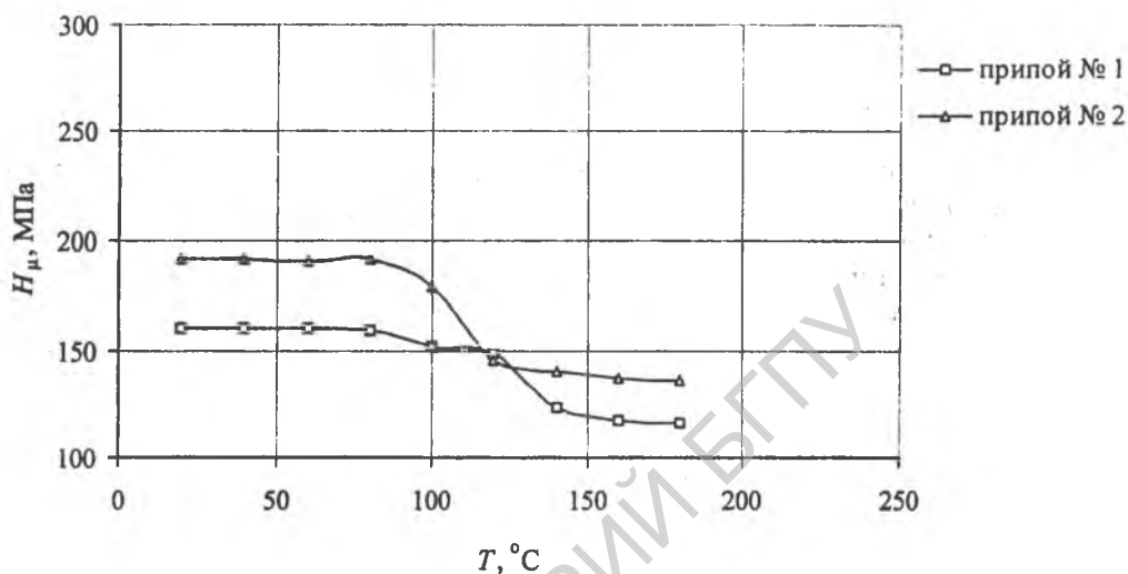
Рис. 3. Изменение микротвердости быстрозатвердевших фольг припоев № 1 и 2 при изохронном отжиге
