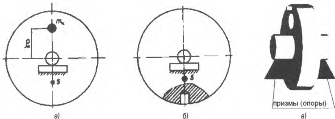
Рисунок 4 – Схема статической балансировки: а – установкой противовеса m_n , б – удалением лишнего материала, в – рисунок, выполненный в AutoCAD
