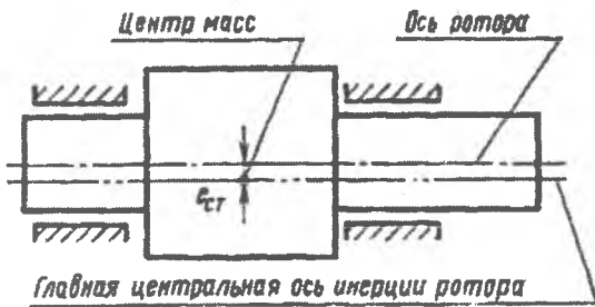
Рисунок 1 – Статическая неуравновешенность ротора
