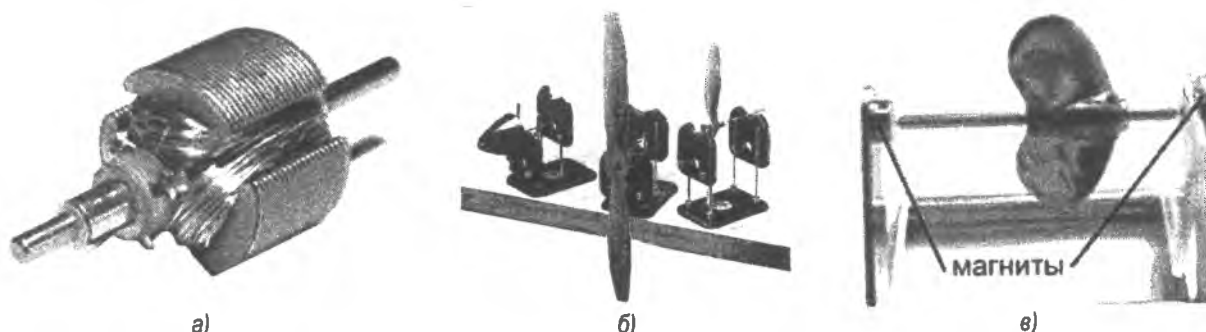
Рисунок 3 – Вращающиеся элементы моделей, испытывающих динамические нагрузки: а) ротор электродвигателя, б) авиамодельный винт, в) судомодельный винт
