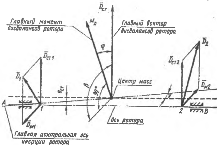
Рисунок 2 – Главный вектор дисбалансов ротора и главный момент дисбалансов ротора
