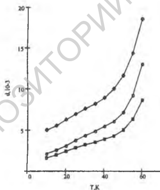
Рисунок 1 – Затухание высокочастотных колебаний как функция температуры в магнитном поле B , Тл: 0(□), 2 (○), 7 (●).
