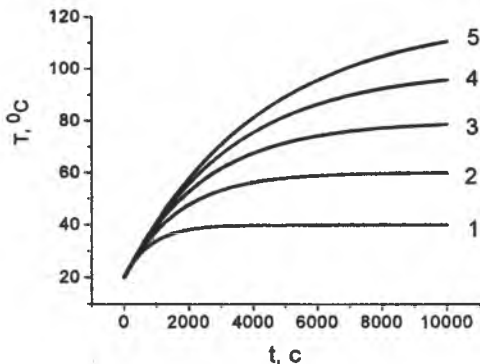
Рисунок 1 – Изменение температуры слоя воды толщиной 10^{-3} м при поглощении мощности 100 \text{ Вт/м}^2 и значениях толщины изолирующего слоя d , м: 0.01 (1), 0.02 (2), 0.03 (3), 0.04 (4), 0.05 (5) и его теплопроводности 0,05 \text{ Вт/м К} .
